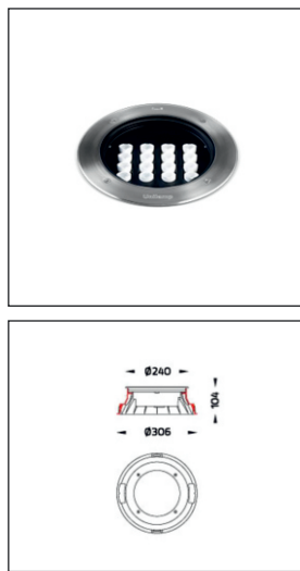
A - Ø306 X H104mm
